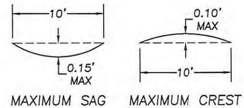
③ APPROACH PROFILE DETAIL SCALE: N.T.S.
