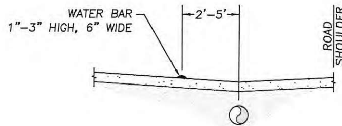
② SECTION A-A SCALE: N.T.S.
