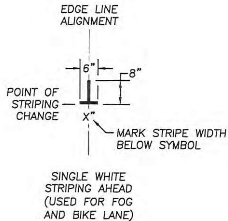
② EDGE LINE STRIPING LAYOUT MARKING SCALE: N.T.S.
