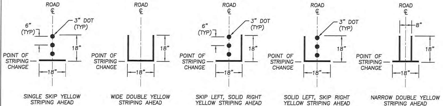
① CENTERLINE STRIPING LAYOUT MARKINGS SCALE: N.T.S.
