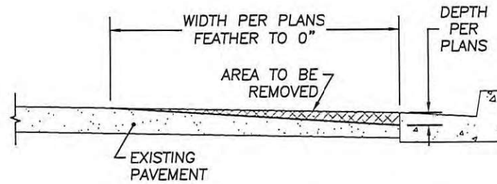
① LONGITUDINAL PAVEMENT REMOVAL DETAIL SCALE: N.T.S.
