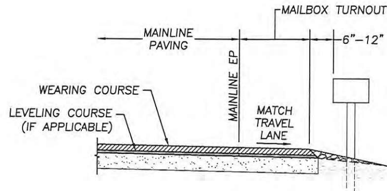
② SECTION A-A SCALE: N.T.S.
