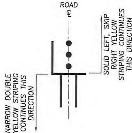
③ EXAMPLE STRIPING LAYOUT MARKING SCALE: N.T.S.
